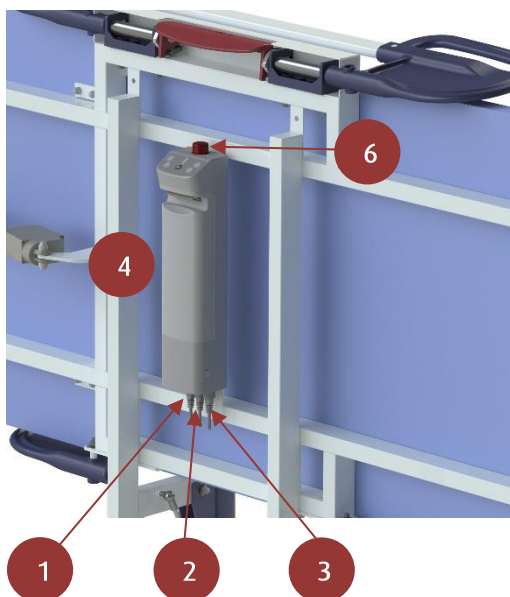
Figuur 4 Elektrische aansluitingen
